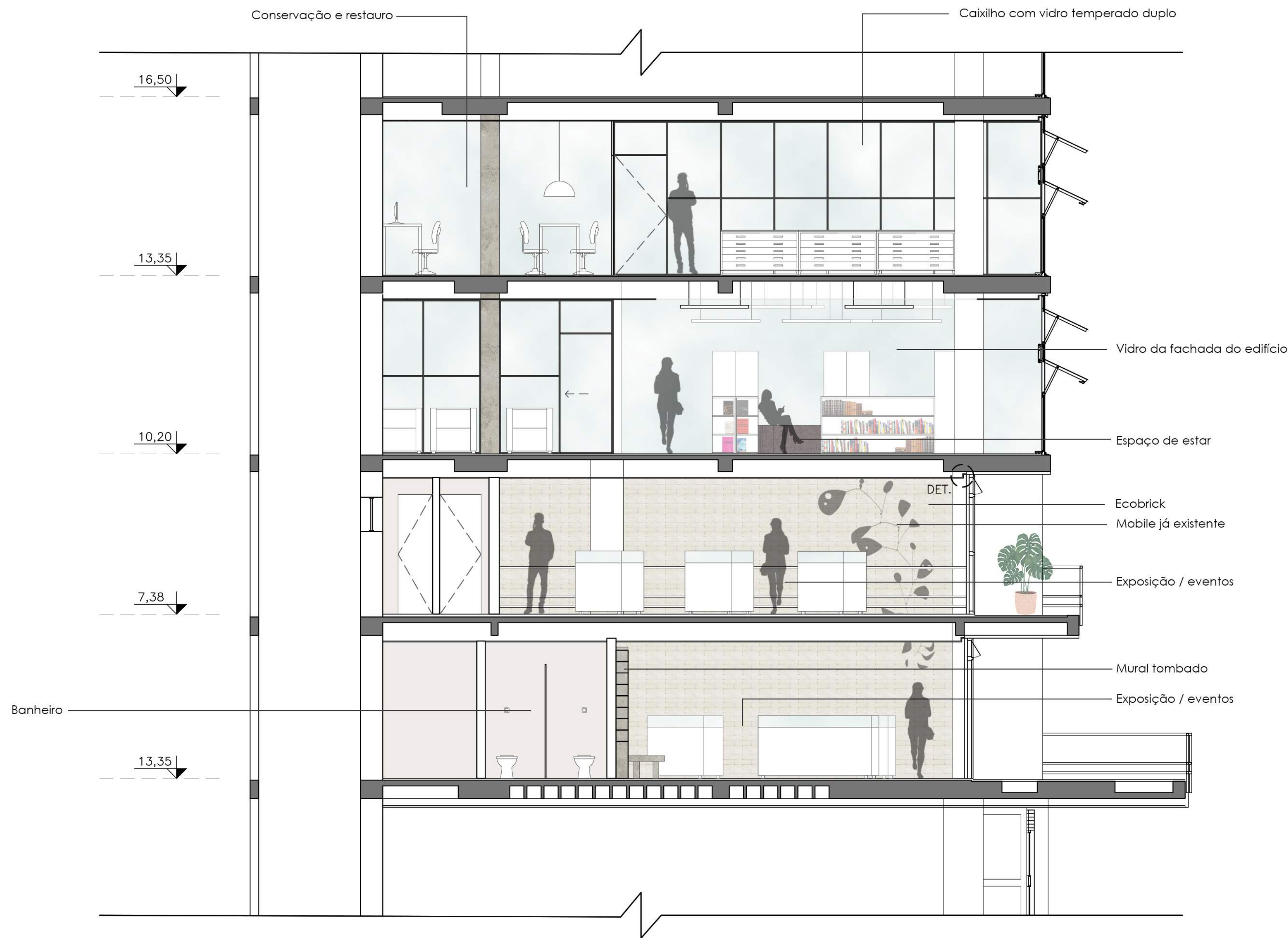
CORTE A-A ESC. 1:50
