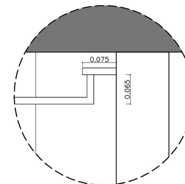
DETALHE — TABICA ESC. 1:5
