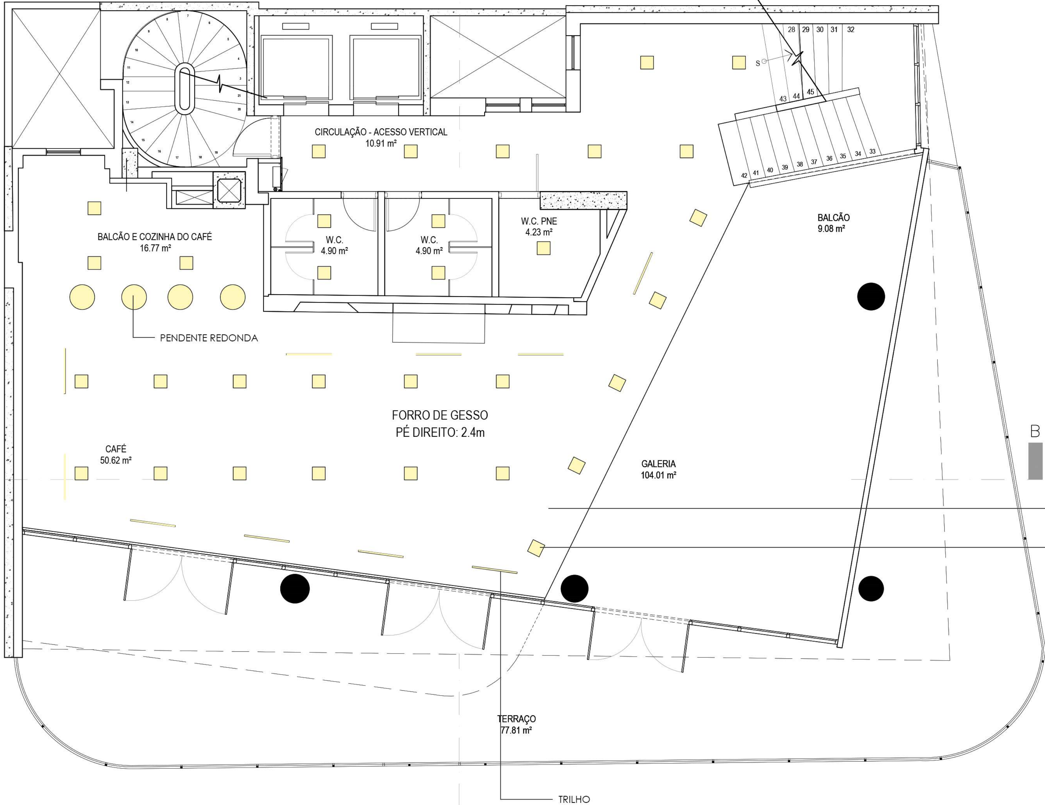
FORRO DO RESTAURANTE 1º PAVIMENTO ESC. 1:50
